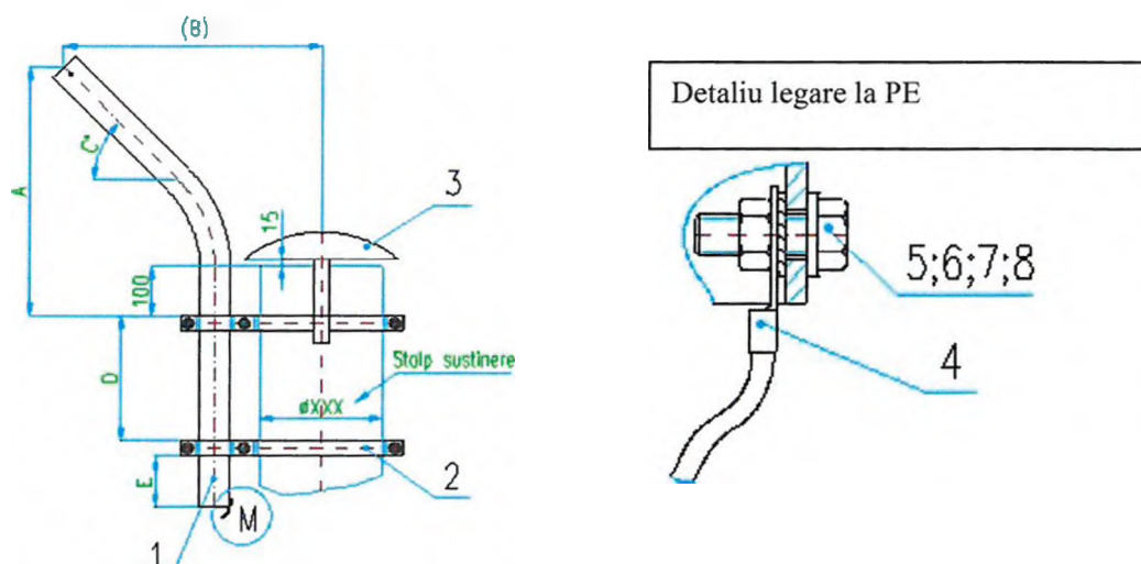
Fig.1-montarea consolei cu coliere pe stâlp: 1 - brat consola ; 2- sistem de prindere; 3- capac stâlp; 4- conductor
