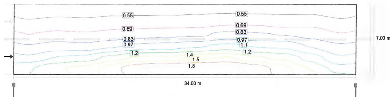
Observator 1: Densitatea luminii la instalația nouă [cd/m²] (Linii Isolux)
